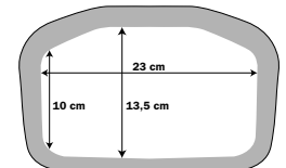
Abmessungen transparentes Deckelfach
